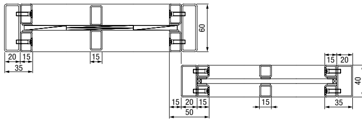
Horizontale doorsnede 1-vleugelige stalen loftdeur met zijdeel
