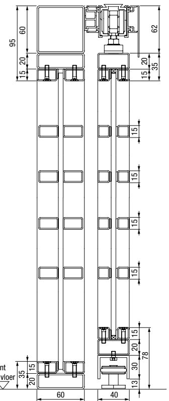
Verticale doorsnede 2-vleugelige stalen loftdeur met zijdelen
