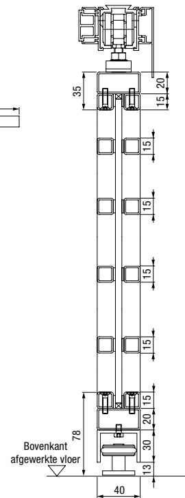
Verticale doorsnede 2-vleugelige stalen loftdeur
